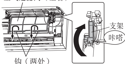
空气过滤网（左右）
