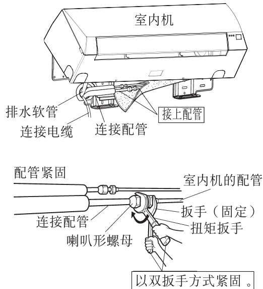
室内机与配管连接（左侧伸出、左后侧伸出时）
