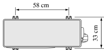
室外机安装孔位置
