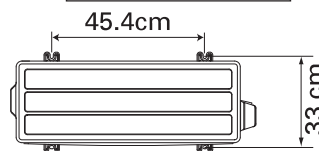
室外机安装孔位置
