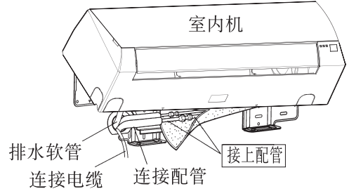
室内机与配管连接（左侧伸出、左后侧伸出时）
