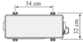
室外机安装孔位置
